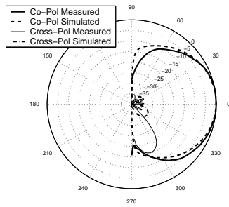
Fig. 7. H-plane Radiation Pattern - 14 GHz Array
