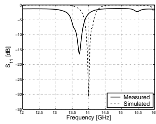
Fig. 4. Return Loss - 14 GHz Array
