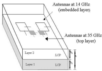
Fig. 1. Multilayer Antenna Array Architecture; h_1 = 8\text{mils} , h_2 = 9\text{mils} , h = 17\text{mils}
