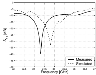
Fig. 5. Return Loss - 35 GHz Array
