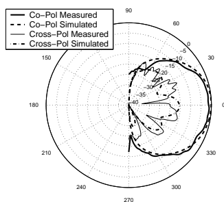
Fig. 9. H-plane Radiation Pattern - 35 GHz Array
